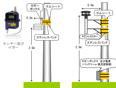
測定機器の設置状況(左:温度計、右:風速計)
