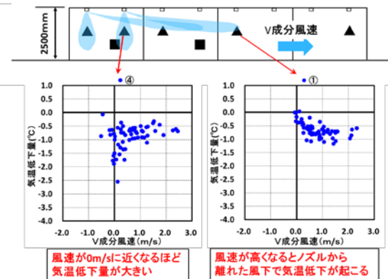
水平風速による風下方向への気温低下領域の拡がり状況
