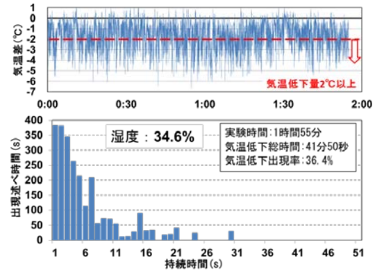
気温低下量の変動(上)と持続時間分布(下)の一例
