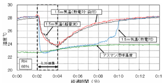
ミスト噴霧環境での気温測定（熱電対では測れていない！）
